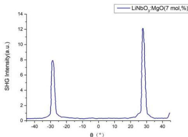
具有I型相位匹配(oo-e)的LiNbO 3 MgO (7mol%) 晶体中SHG强度的角度依赖性
