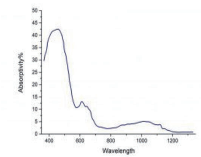
Cr 4+ : YAG吸收光谱
